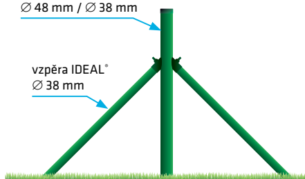
sloupek IDEAL® Ø 48 mm / Ø 38 mm
